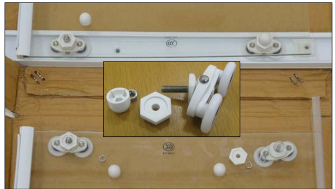
Рис. 54. Установка роликов дверей
