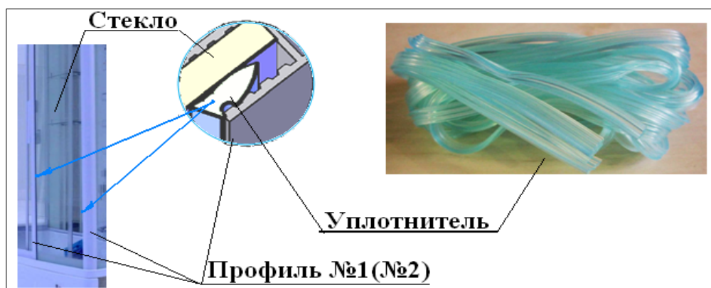
Рис.60. Установка уплотнителей переднего стекла.
