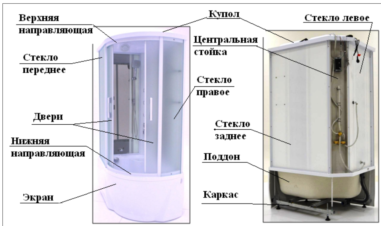
Рис.2. Устройство душевой кабины “Сириус”
