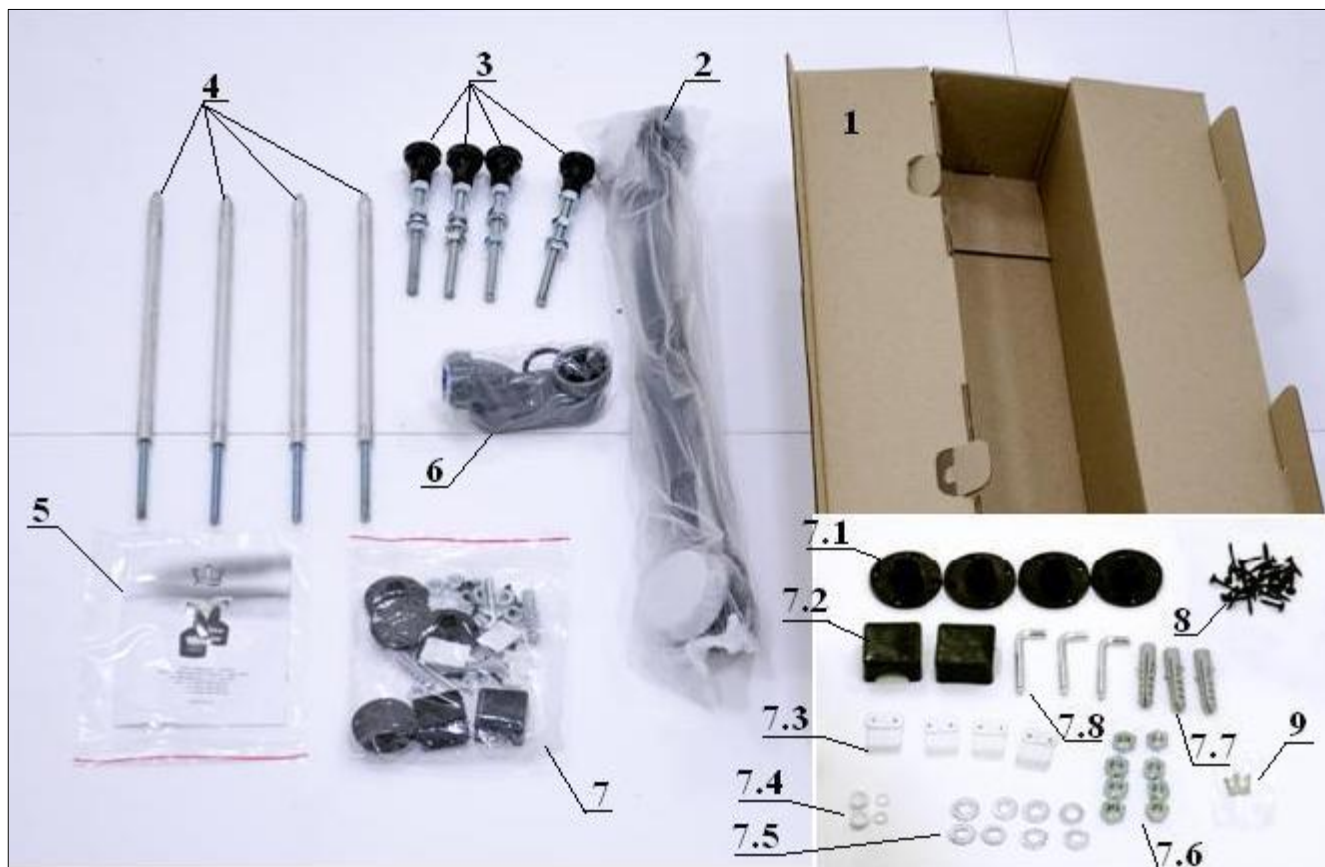
Рис. 66. Установочный комплект душевой кабины “Сириус”
