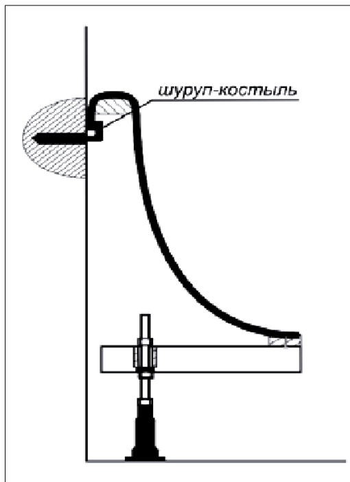
Рис. 64. Соединение со стеной
