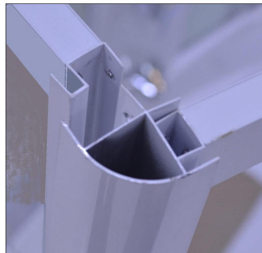
Рис. 41. Совмещение профилей и стойки.
