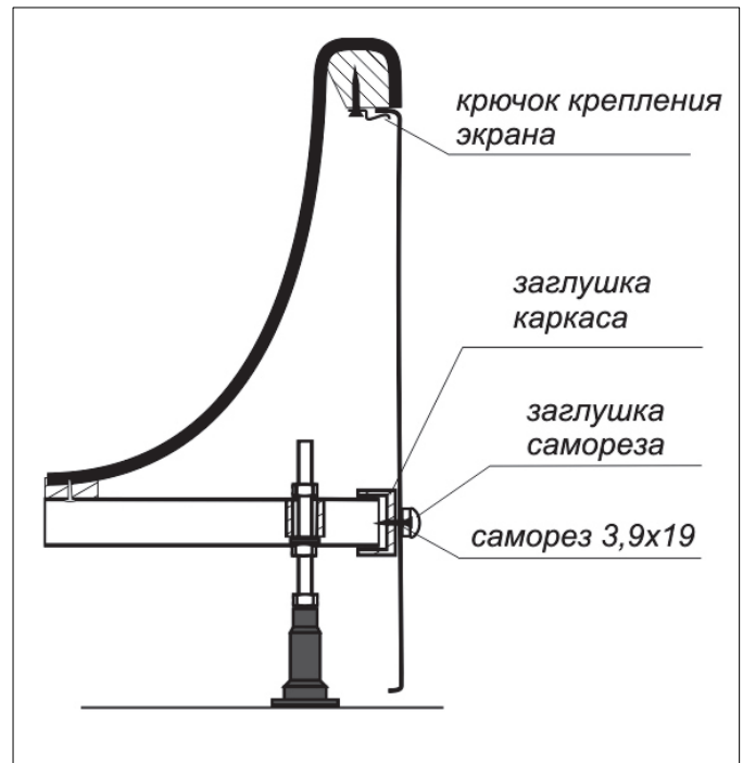
Рис. 65. Установка экранов
