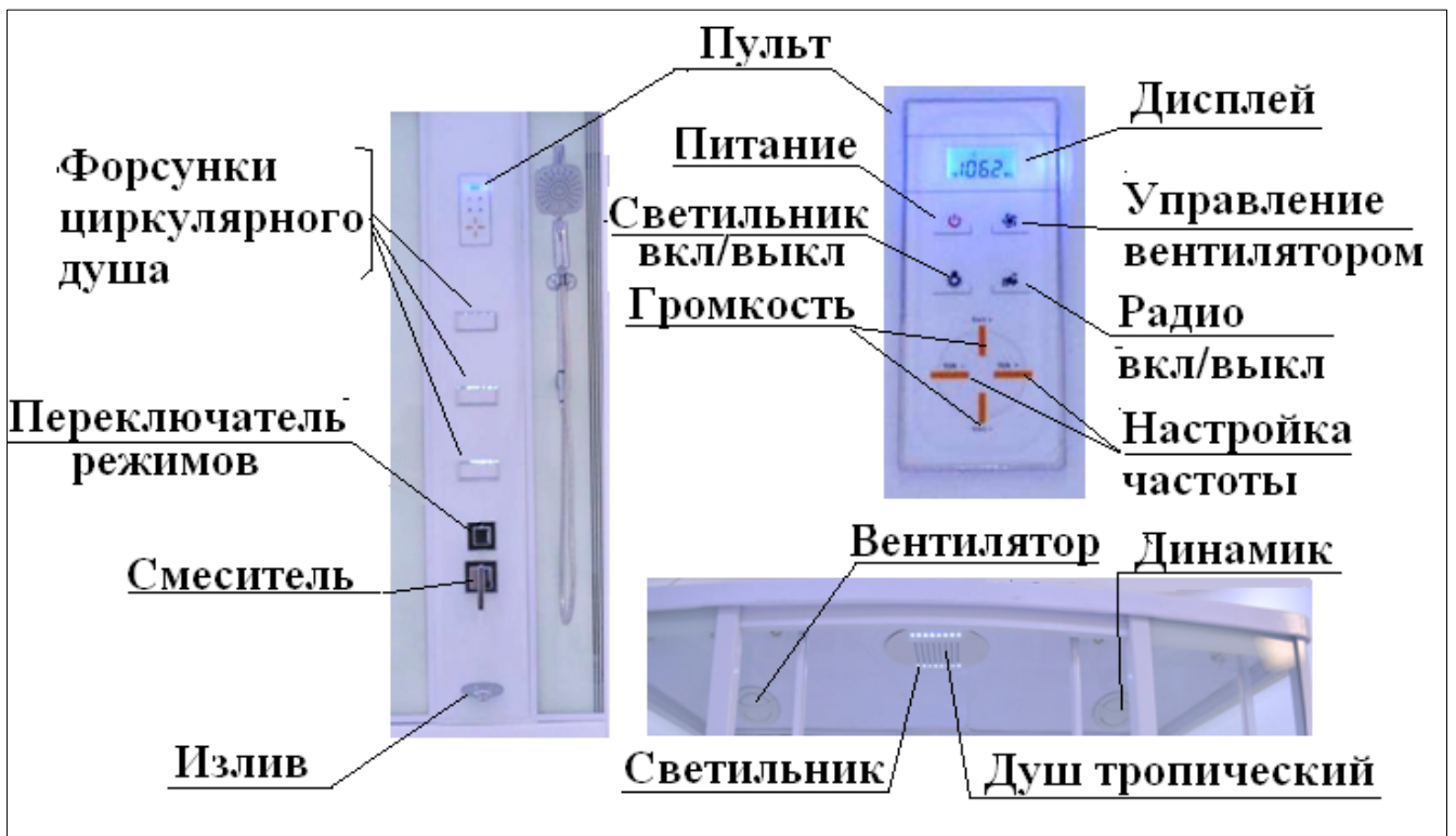
Рис. 62. Органы управления оборудованием
