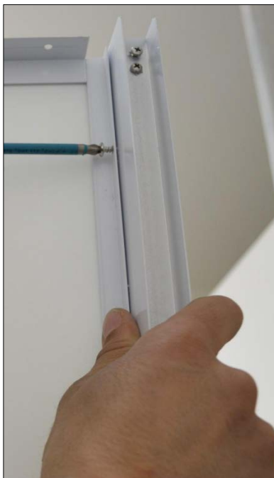
Рис. 34. Соединение стекол
