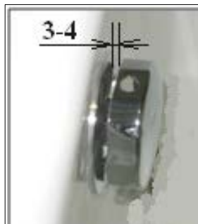
Рис. 16.1. Установка зазора
