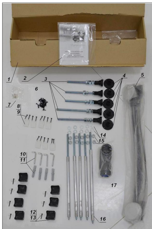
Рис.6. Установочный комплект
